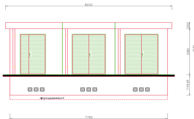
ФАСАДА 2-2
