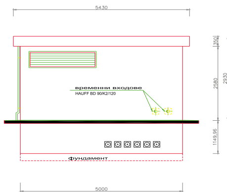
ФАСАДА 1-1
